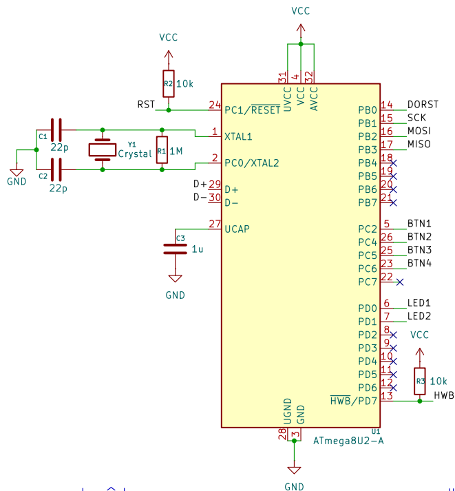
Microcontrôleur
