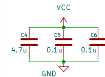
CONDENSATEUR DE DECOUPLAGE
