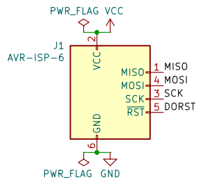
Connecteur ISP (Femelle)
