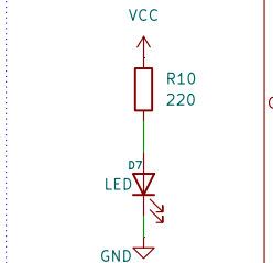
LED ETAT D'ALIMENTATION
