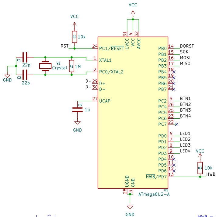
Microcontrôleur
