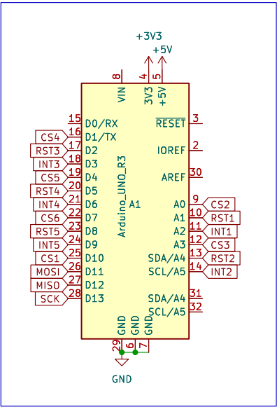
Bouclier Arduino Uno
