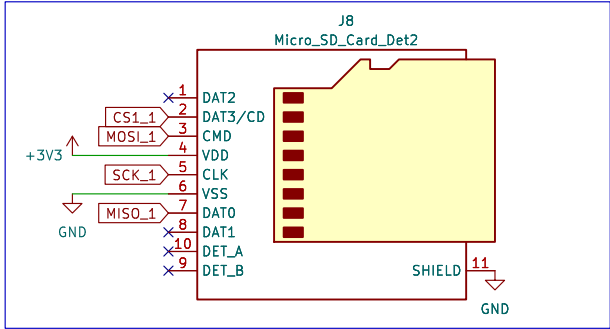
Lecteur SD
