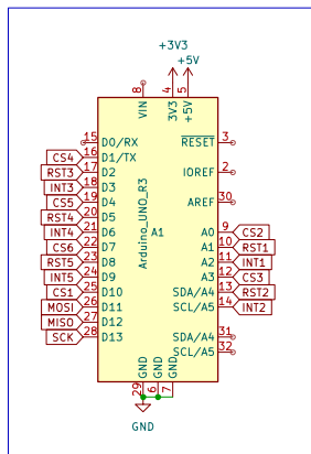
Bouclier Arduino Uno
