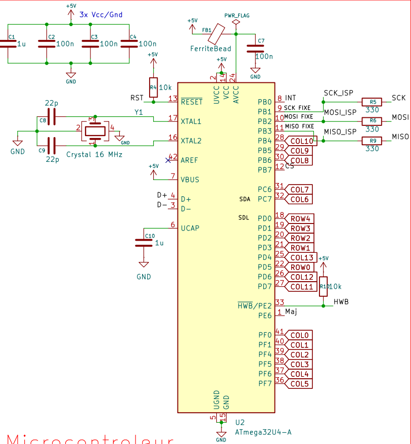
Microcontrôleur
