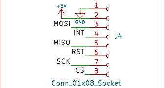
Connecteur Carte Mere
