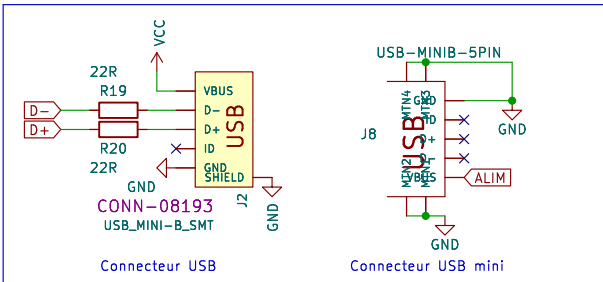
Connecteur USB
