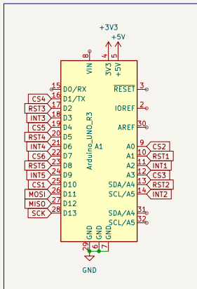
Bouclier Arduino Uno
